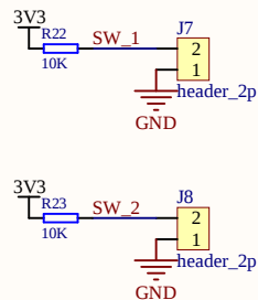
微动开关接口, XH2.54, 2P
